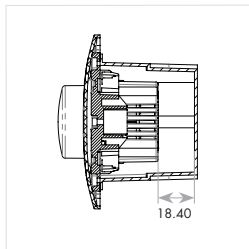
חתך צד
